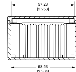
SECTION D-D
