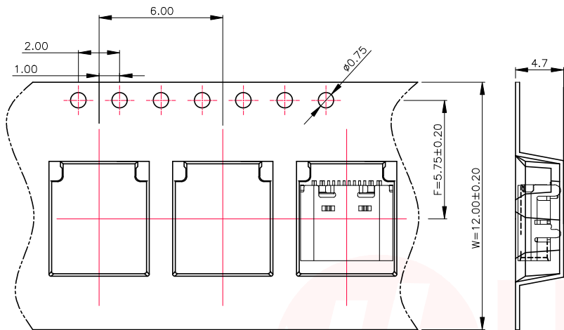
① 产品入载带示意图
