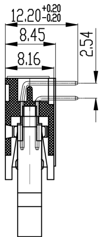
弯针
