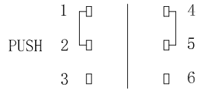
电路简示图
