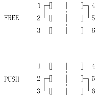
电路简示图
