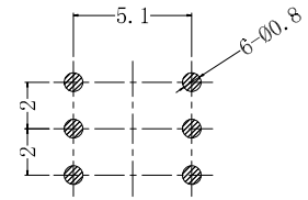
PCB参考图
