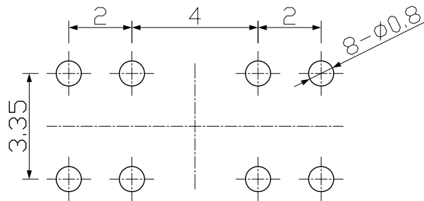
印制线路板
