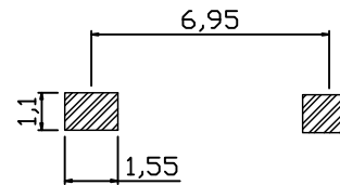
PCB. 焊接图
