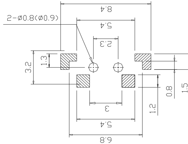
PCB. 焊接图
