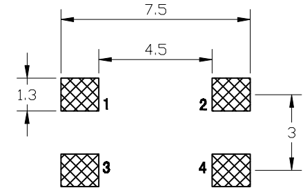
安装尺寸 (从焊锡面看)
