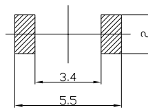
安装参考尺寸
