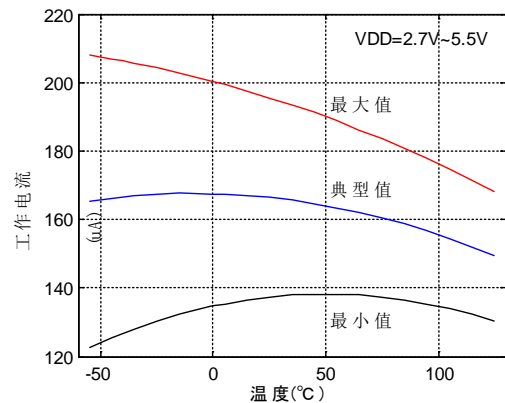
图 16. 测温工作电流
