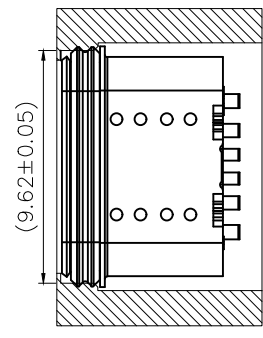
组装示意图
