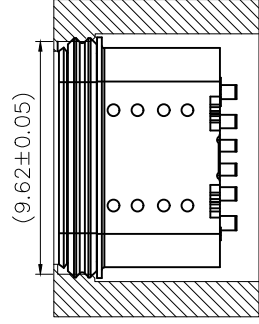
组装示意图
