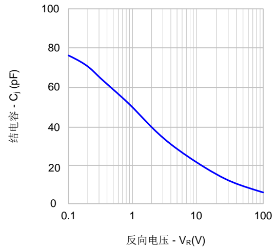
图2. 结电容特性
