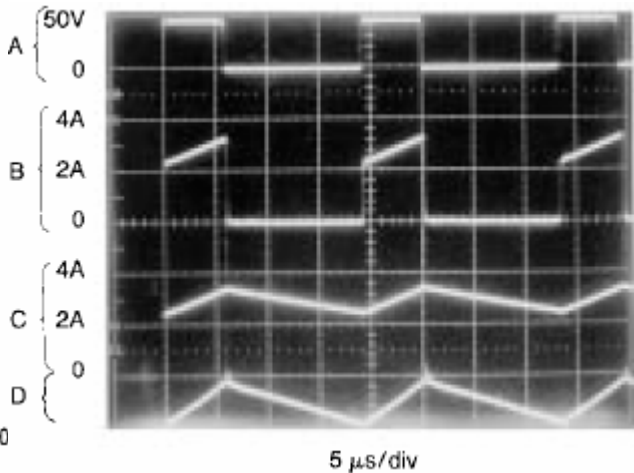
开关波形
