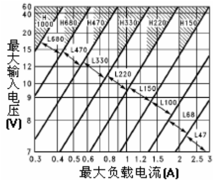
图 5. HYM2576(HV)-5.0
