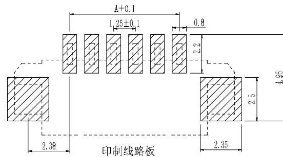
印制线路板
