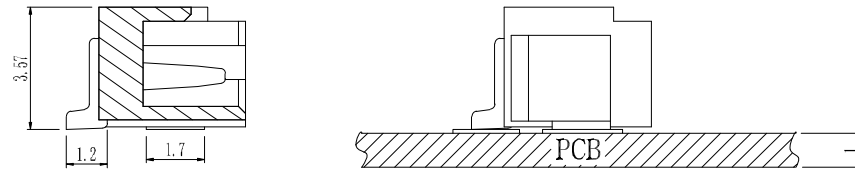
截面 A-A
