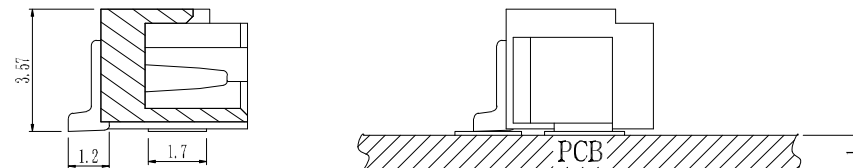
截面 A-A
