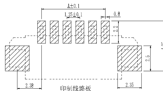
印制线路板
