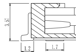
截面 A-A
