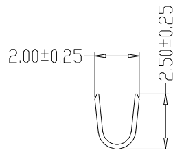
SEC:B-B
