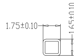
SEC:D-D
