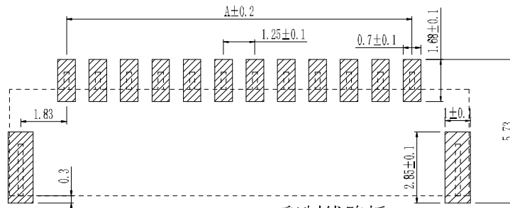
印制线路板
