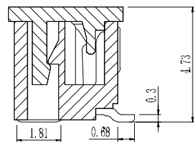
截面 A-A
