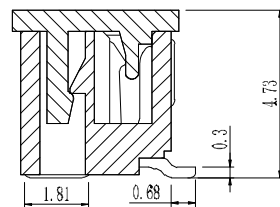
截面 A-A
