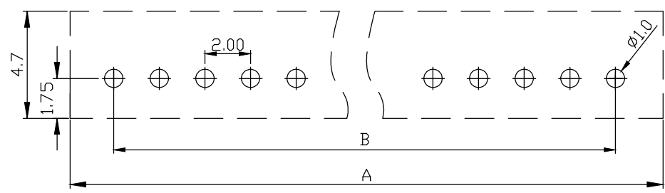
PCB参考图
