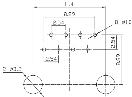
PCB参考图
