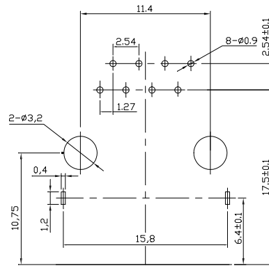
P. C. B参考图
