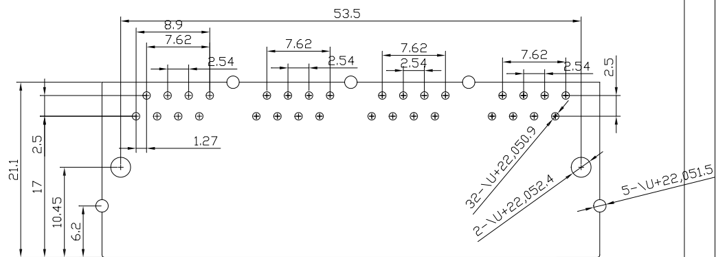
PCB参考图
