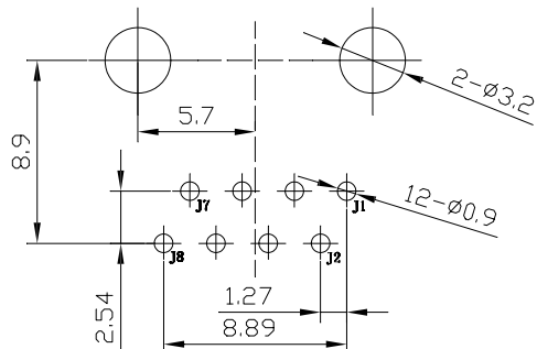
P.C.B参考图 (建议板后1.6mm)
