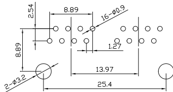
P.C.B参考图
