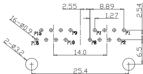
P.C.B参考图
