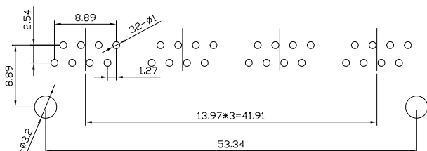
P.C.B参考图
