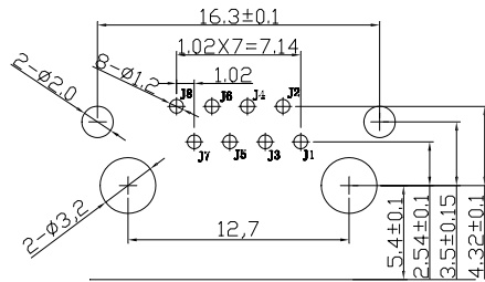
P.C.B参考图
