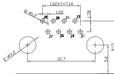
P.C.B参考图
