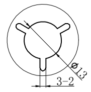
DETAIL: A 10:1
