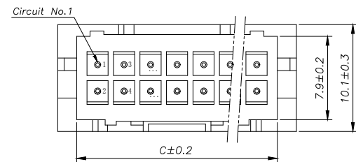
2x2~2x8Pin
