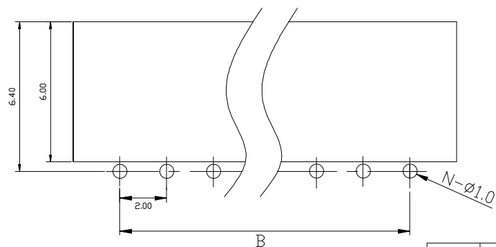
PCB参考图
