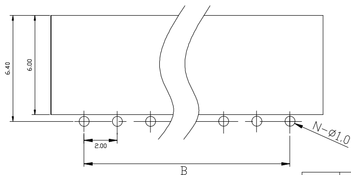
PCB参考图
