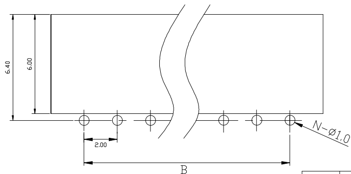
PCB参考图
