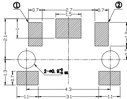
P.C.B.Land Pattern
