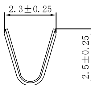
A-A旋转
