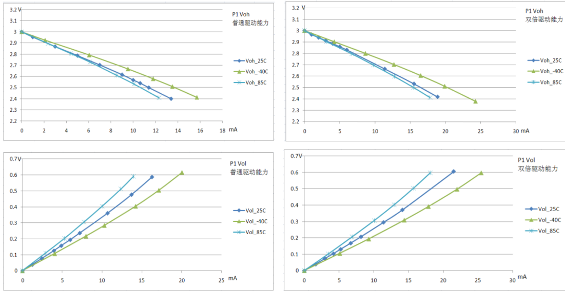
图 3.4 端口 P1 V OH /V OL 实测曲线
