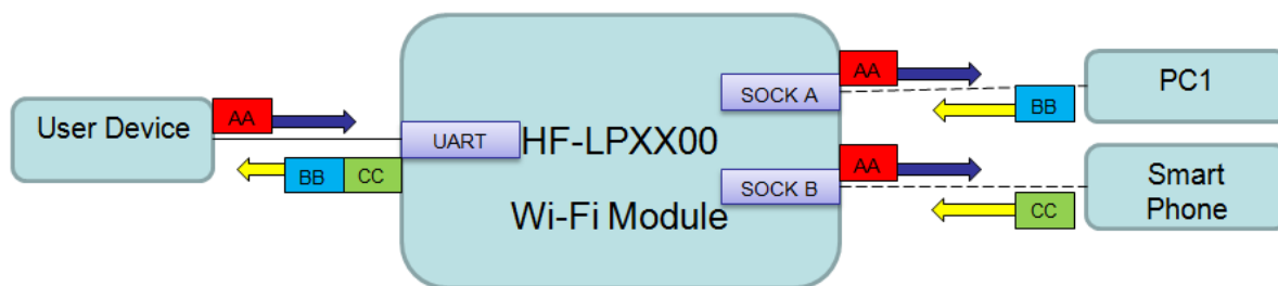
Figure 19. 双 Socket 数据流向示意图
