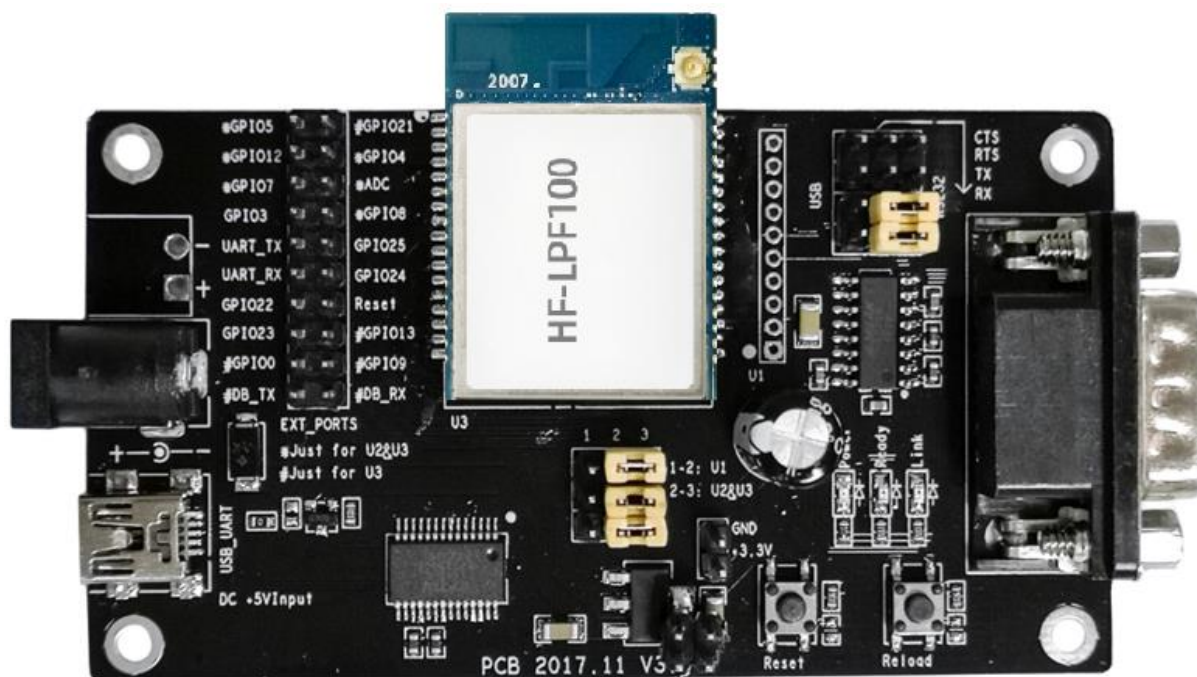
Figure 5. HF-LPF100 开发板
