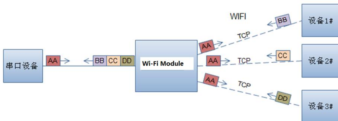
Figure 21. 多 TCP 链接数据传输图示
