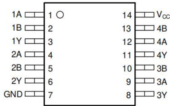
DIP14/SOP14/TSSOP14
