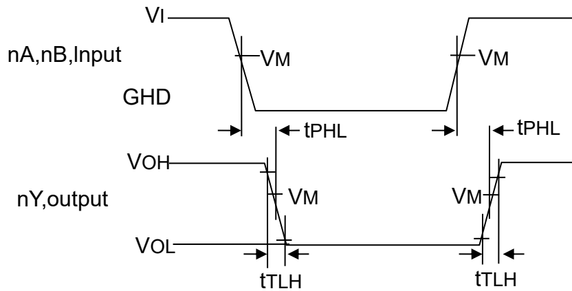
图 3、数据输入 (1An,2An) 到数据输出(1Yn, 2Yn)传输延迟时和输出 (nYn) 转换时间波形
