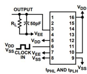
Fig. 7 传播延迟-使能输入 to 开关输出
