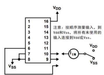
Fig. 4 输入电流
