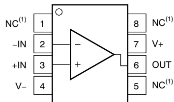
封装：HGV333 8 引脚小外形尺寸集成电路 (SOP) 封装 俯视图
