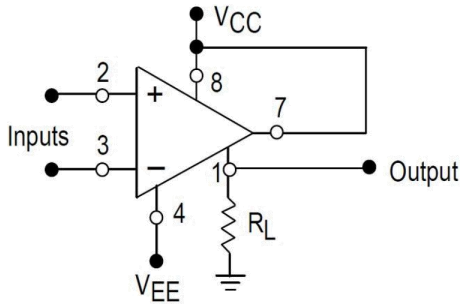
(当 GND 作为输出时, 输入极性反转)
