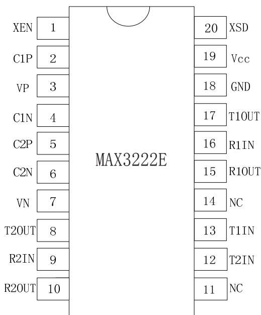
20-pin SSOP/TSSOP
