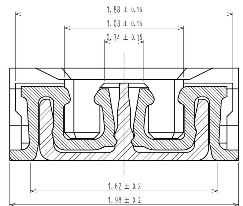
A-A (50:1)
