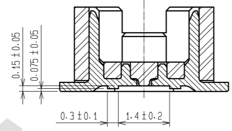
F-F (10:1)
