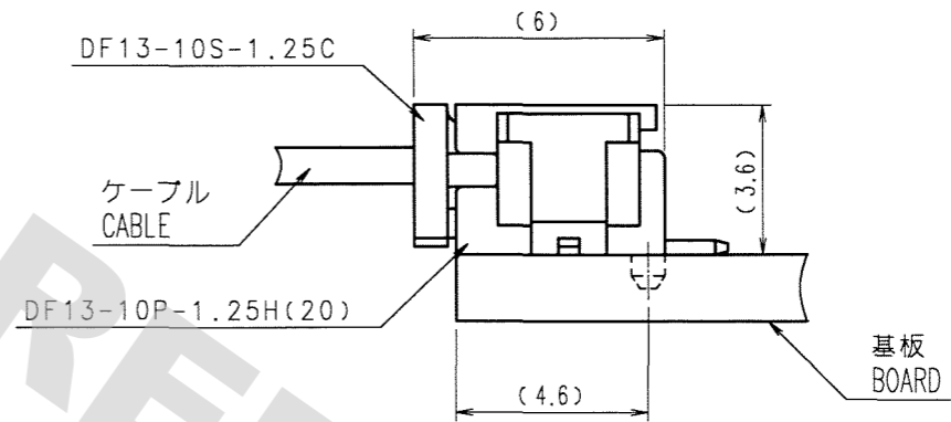
ソケット嵌合図 MATED CONNECTORS
