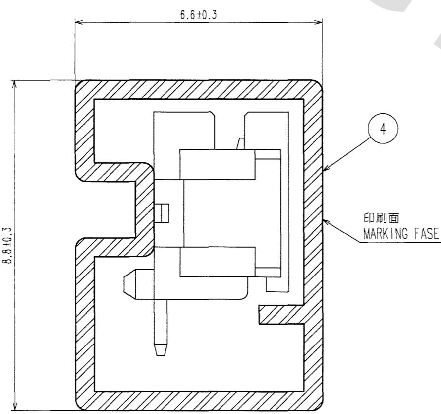
A-A (10:1)
